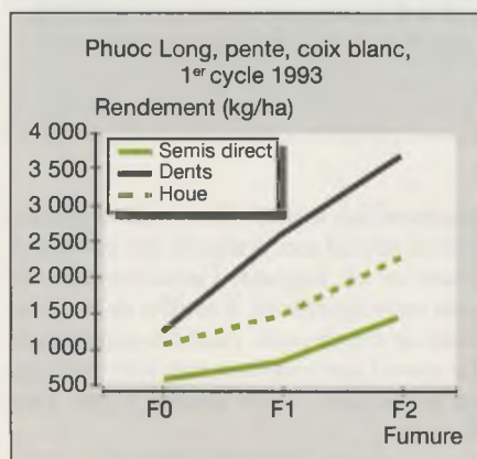
Figure 6. Effets des différents modes de travail du sol et de trois niveaux de fumure sur le rendement du coix blanc sur les sols des flancs dégradés des hautes collines basaltiques.
