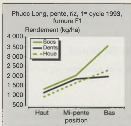
Figure 4. Effets des différents modes de travail du sol et de la localisation sur la pente sur le rendement du riz pluvial sur les sols des flancs dégradés des hautes collines basaltiques.
