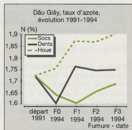
Figure 8. Evolution de la teneur en azote du sol en fonction du mode de travail du sol et du niveau de fumure, sur les sols des basses collines basaltiques.
