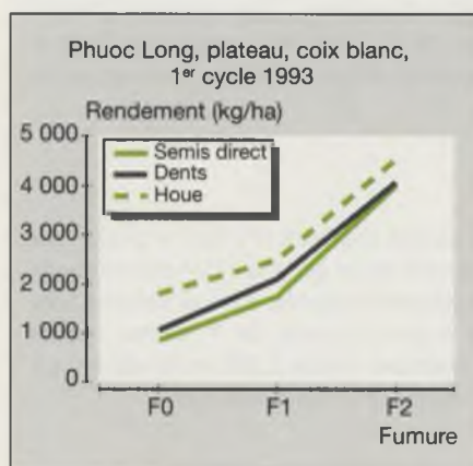
Figure 5. Effets des différents modes de travail du sol et de trois niveaux de fumure sur le rendement du coix blanc sur les sols de plateaux des hautes collines basaltiques.
