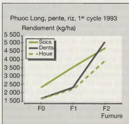
Figure 3. Effets des différents modes de travail du sol et de trois niveaux de fumure sur le rendement du riz pluvial sur les sols des flancs dégradés des hautes collines basaltiques.
