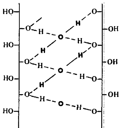
Cellulose « hydratée »
