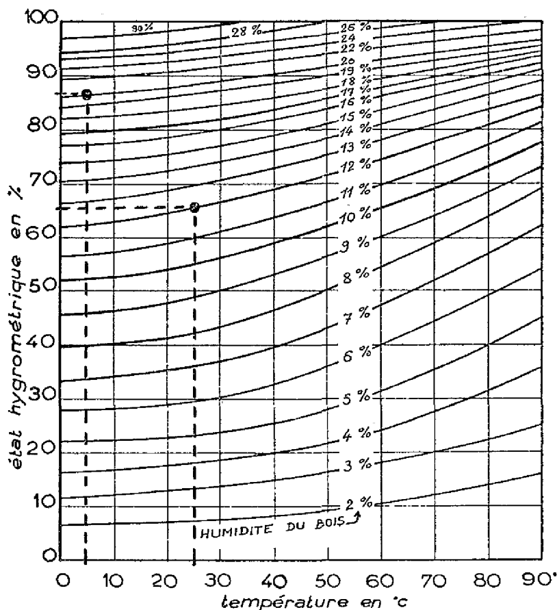
FIG. 1. — Courbes d'équilibre hygroscopique du bois.
