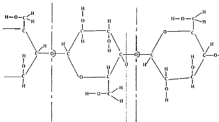
Molécule de cellulose
