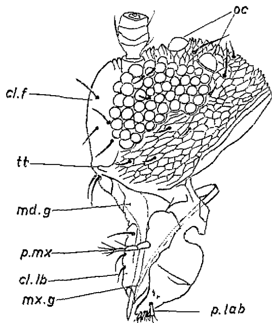
Fig. 3. — Caliothrips helini Hood : Tête vue de profil. oc. : ocelles. cl. f. : clypeo front. tt. : tentorium. md. g. : mandibule gauche. p. mx : palpe maxillaire. cl. lb. : clypeo labre. mx. g. : maxille gauche. p. lab. : palpe labial.
