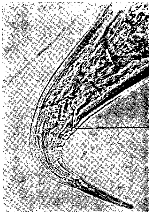
Fig. n° 2. — Extrémité caudale (× 60).
