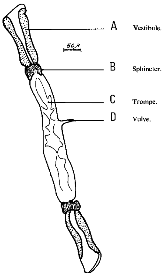
Fig. n° 1. — Ovojecteur.
