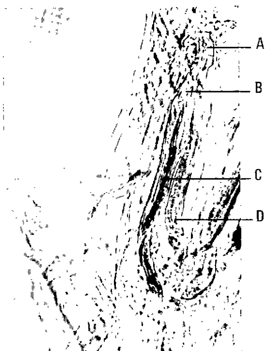
Fig. n° 1. — Spicules ( \times 570 ).
