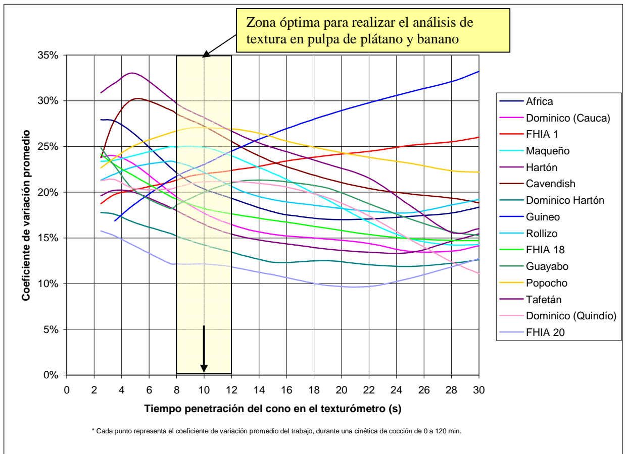
Fig. 1 Coeficientes de variación del trabajo de penetración en el análisis de textura durante los estudios de cocción en agua de musáceas colombianas
