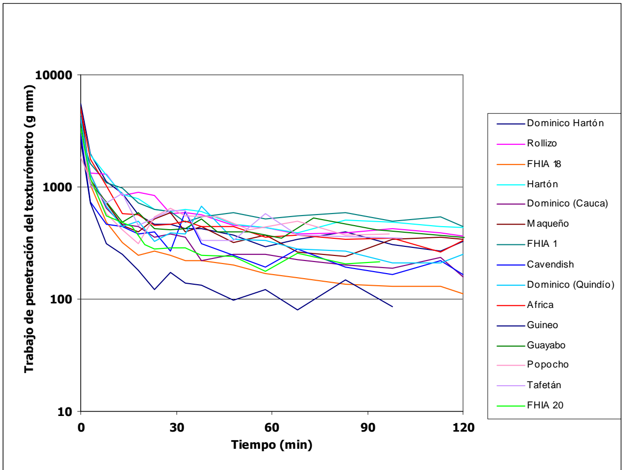
Fig. 2 Modificación de la firmeza durante la cocción en agua de musáceas colombianas
