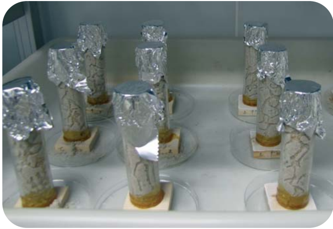
Essai de résistance aux termites. © N. Leménager, Cirad
