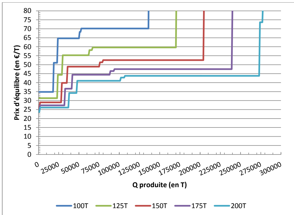
Figure 4. Courbe d'offre inverse de la canne fibre pour différents niveaux de rendement de la canne fibre.
