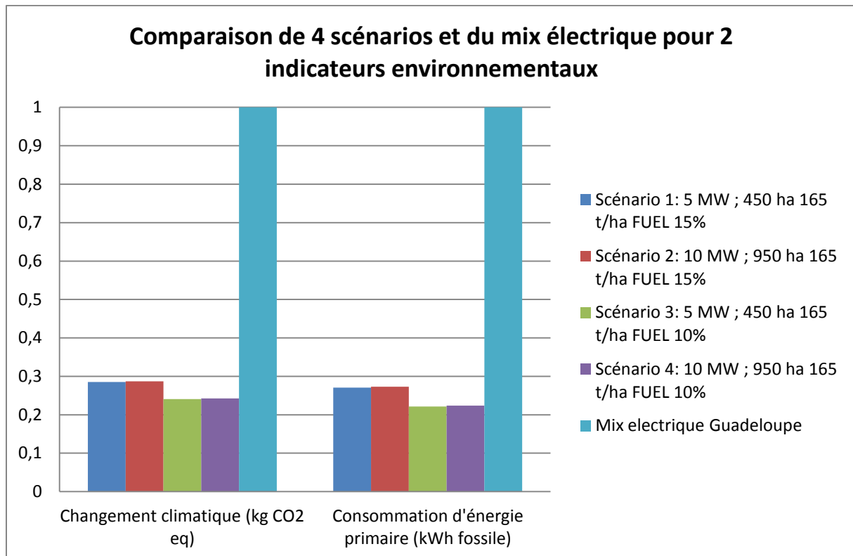
Figure 5 : Exemple de résultats relatifs à 4 scénarios et au mix électrique Guadeloupe estimés sur la base de 2 indicateurs de l'ACV. Les scénarios 3 et 4 sont des variantes des scénarios 1 et 2 à 10% de fuel au lieu de 15%.
