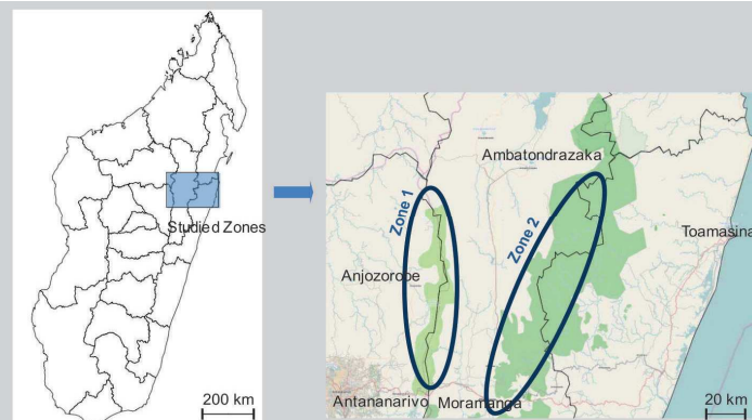
Figure 1. Zones étudiées : Zone 1, Corridor forestier de l'Angavo ; Zone 2, corridor forestier de l'Ankai
