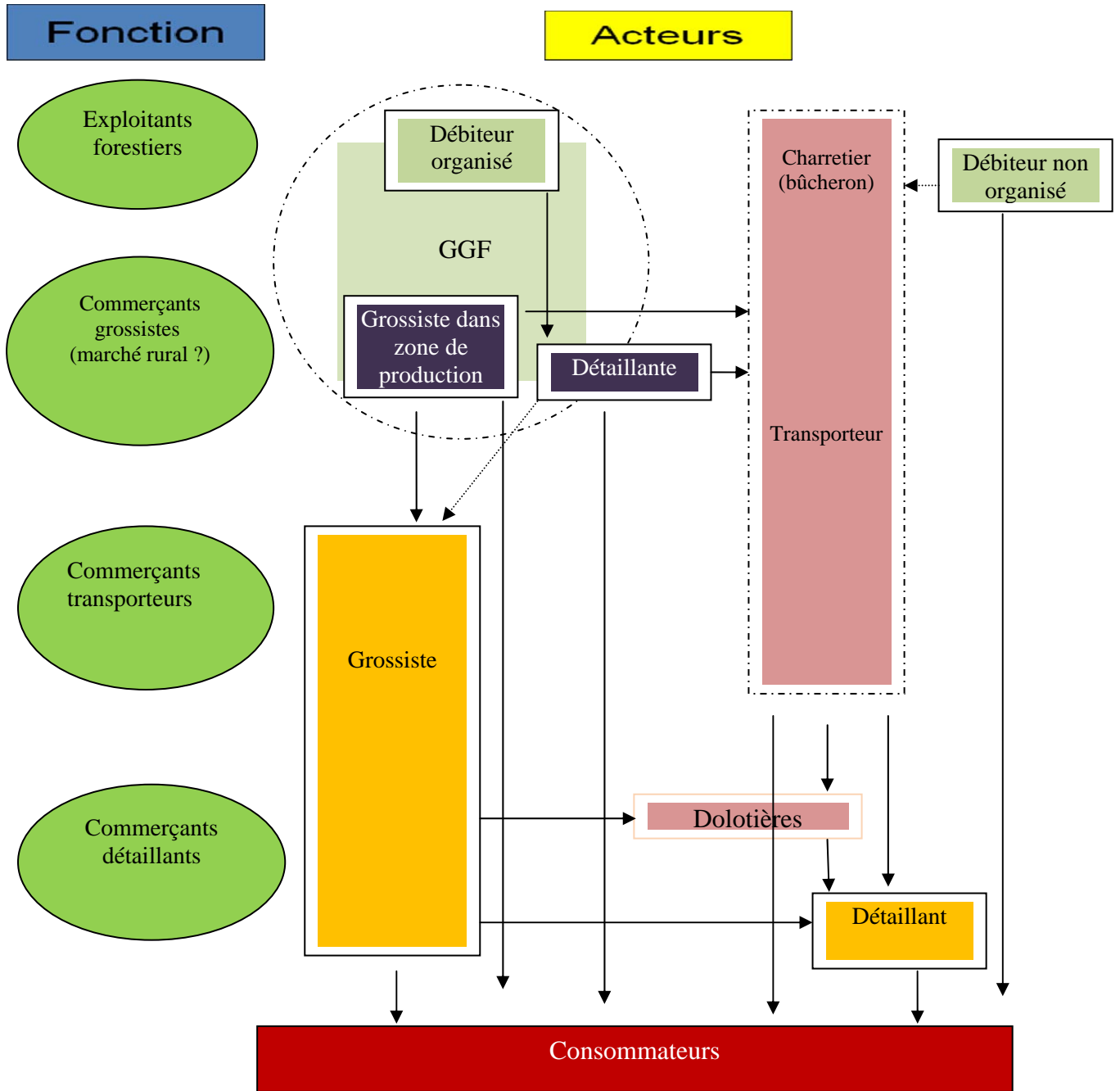
Figure 1 : Relations entre les agents de la sous-filière bois de chauffe
