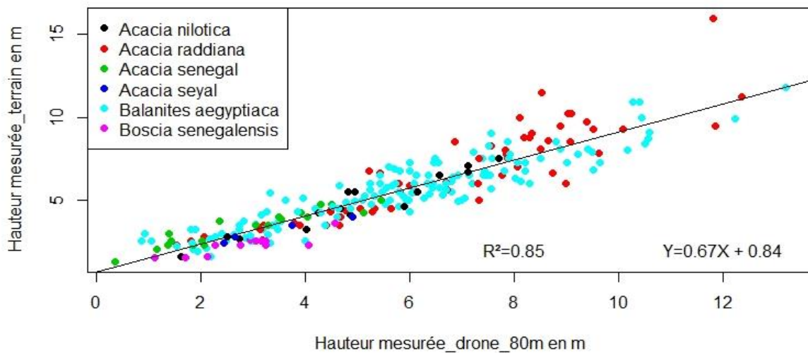
Figure 7: Régression linéaire sur les mesures de hauteur à 80 m
