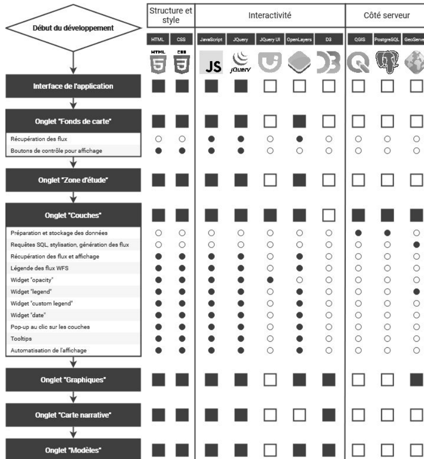
Figure 2. Principales étapes du développement de l'application et technologies mobilisées (source : les auteurs)
